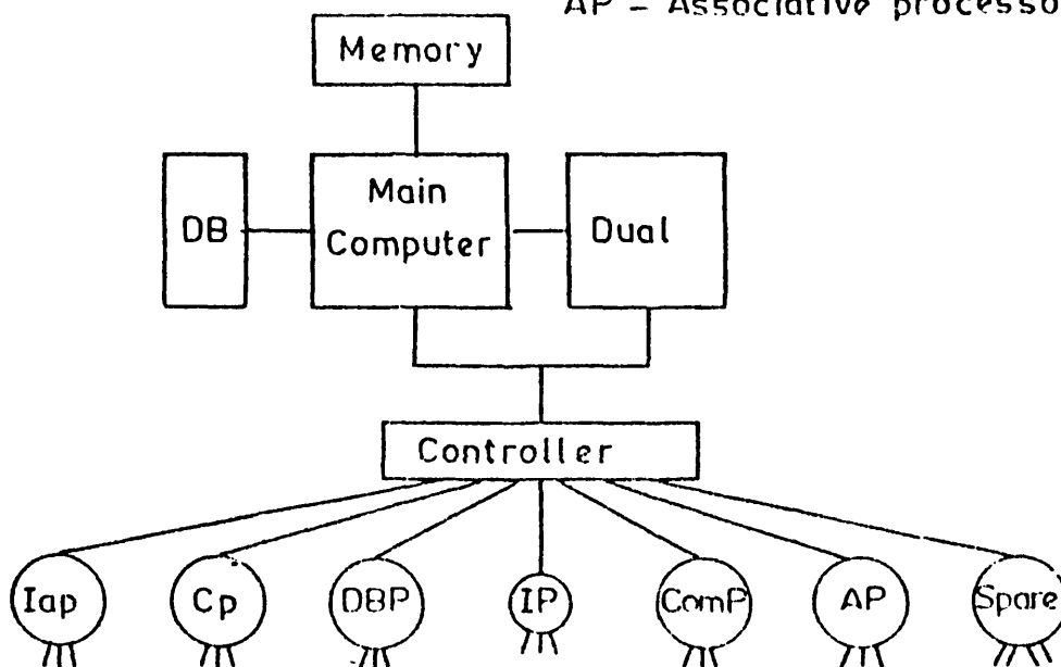
Fig. 4 (d) - A star network configuration for the central dispatch centre
